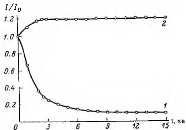
Рис. 1. Графік залежності зміни величини I/I_0 від часу опромінення електронним пучком (1 – F, 2 – Ca).
