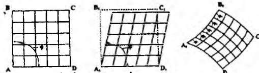
Мал. 4. Зміна кута між системою ниток у тканині під дією зовнішніх сил.
