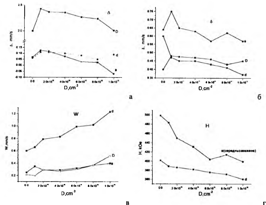
Рис. 1. Залежність параметрів КЕМ спектрів іонно-імплантованих плівок ЗІГ від дози опромінення.
